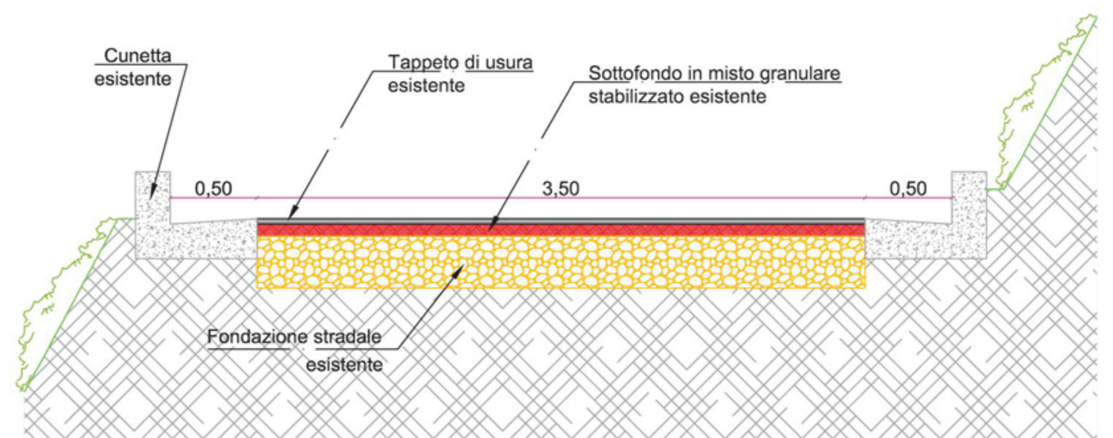
SEZIONE "A-A" (stato dei luoghi) da picchetto 1 a 6 Scala 1:25
