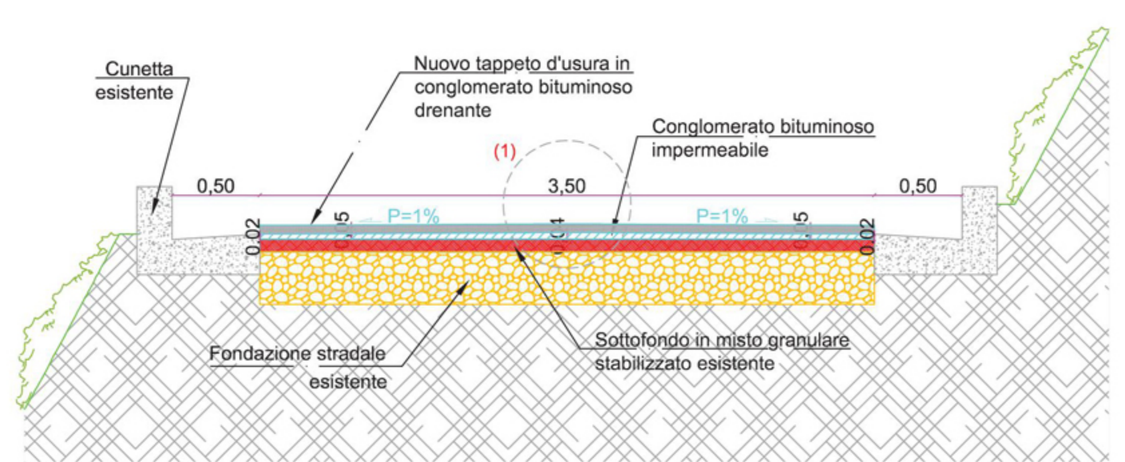
SEZIONE "A-A" (stato di progetto) da picchetto 1 a 6 Scala 1:25
