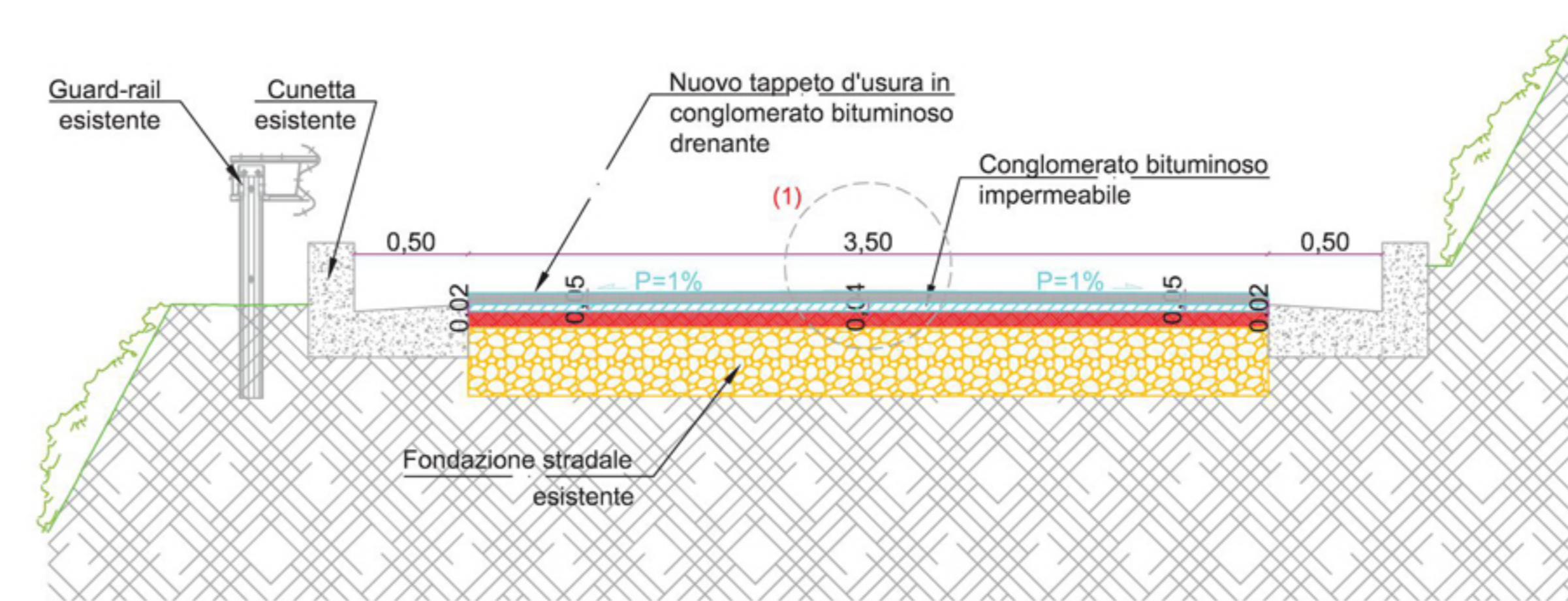
SEZIONE "B-B" (stato di progetto) da picchetto 6 a 26 Scala 1:25
