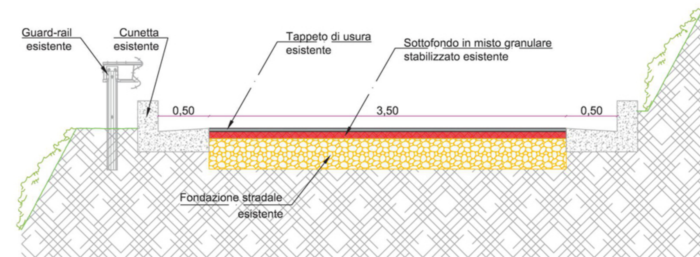
SEZIONE "B-B" (stato dei luoghi) da picchetto 6 a 26 Scala 1:25
