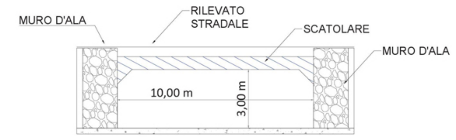
PROSPETTO LATO MONTE
